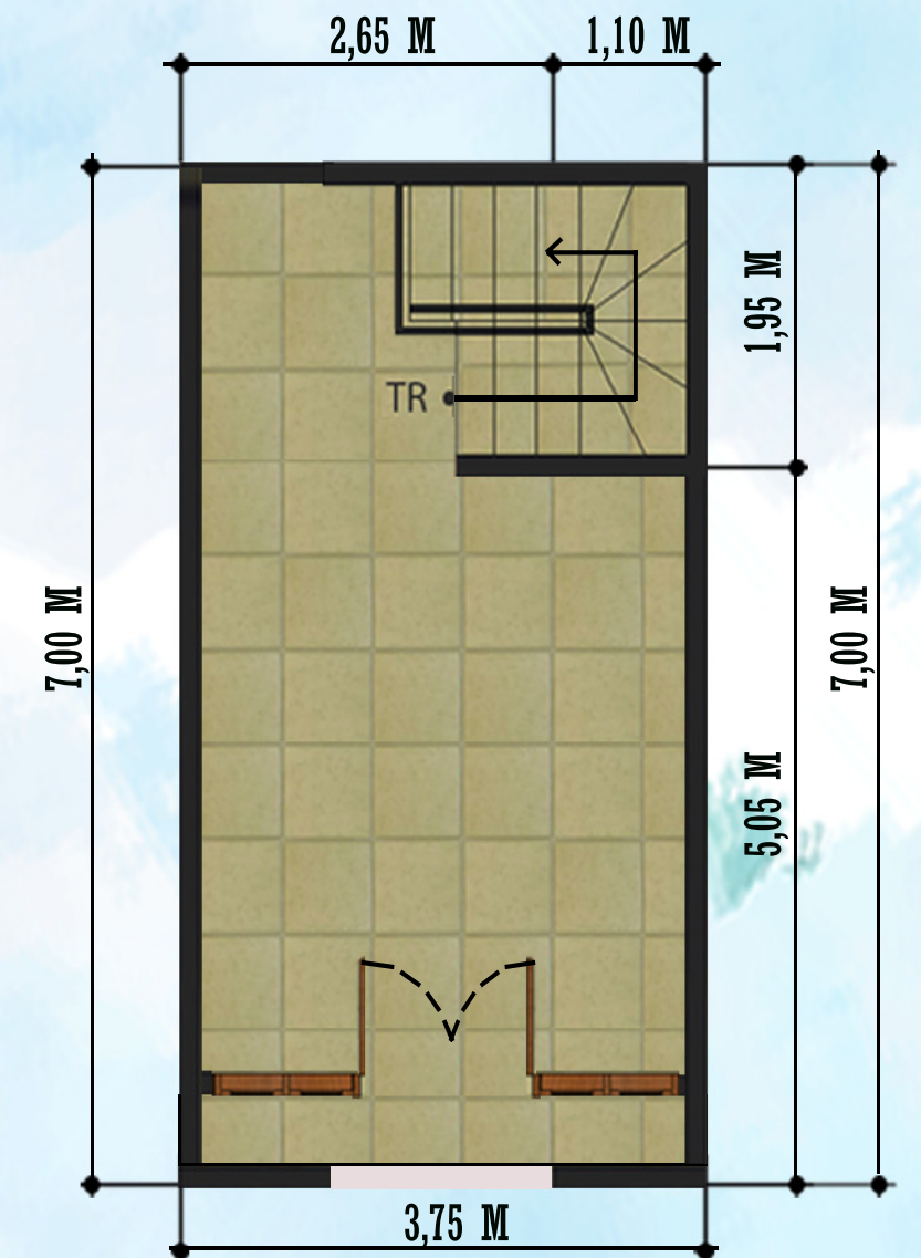
LANTAI 2
