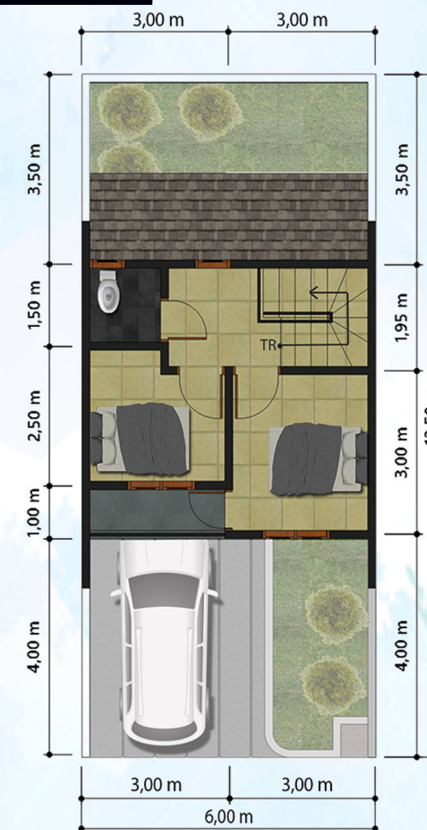
LANTAI 2
